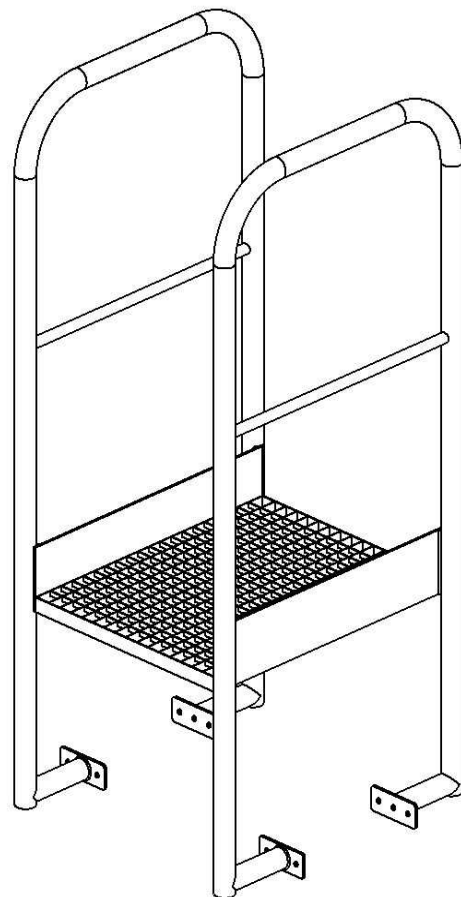
Übersteigbügel mit Trittpläche Form C
